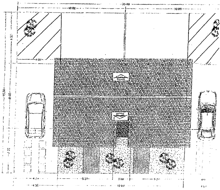
CUBIERTA E IMPLANTACION GENERAL Escala 1:100
