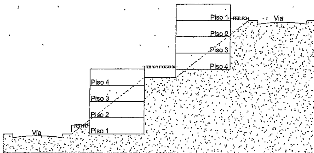
EDIFICACION EN LOTE - B4 a B7
