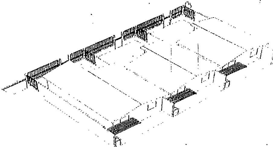
VISTA ISOMETRICA SE
