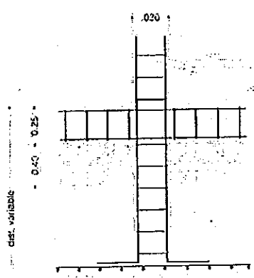
DETALLE DE PLINTO
